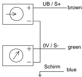
Cable outlet
